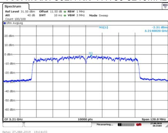
Test Mode: 802.11ac VHT80 5210MHz
