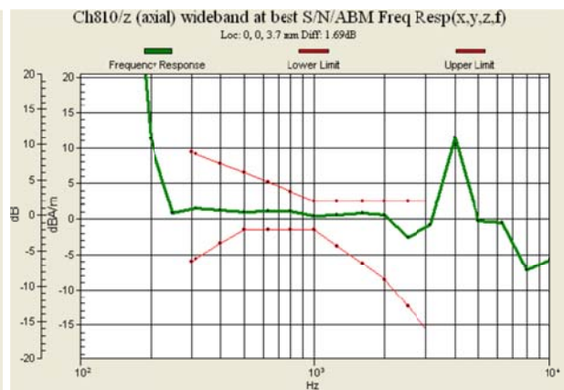
Fig 7.6 GSM1900 Ch810
