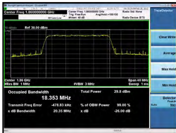
NR n25 16QAM 20MHz CH-Middle
