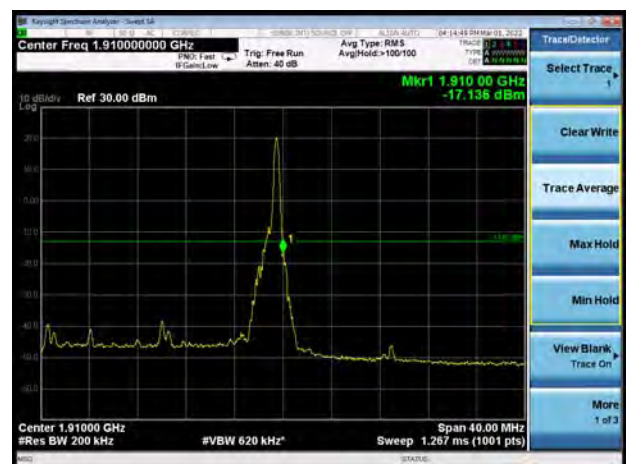
DC_12A_n2A QPSK 20MHz CH-High 1RB
