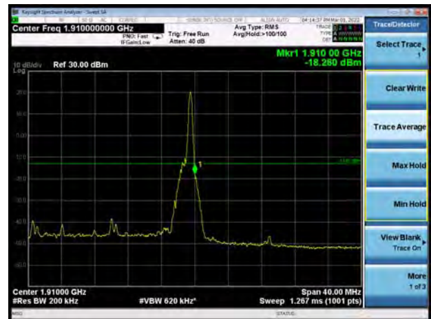
DC_12A_n2A P1/2 BPSK 20MHz CH-High 100%RB
