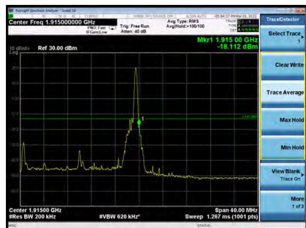
NR n25 QPSK 20MHz CH-High 1RB
