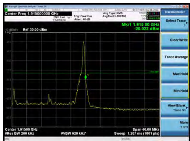
DC_66A_n25A QPSK 20MHz CH-High 1RB
