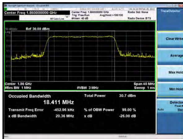
NR n25 P1/2 BPSK 20MHz CH-Middle
