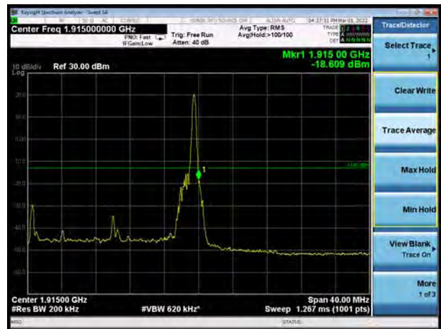
DC_66A_n25A P1/2 BPSK 20MHz CH-High 100%RB
