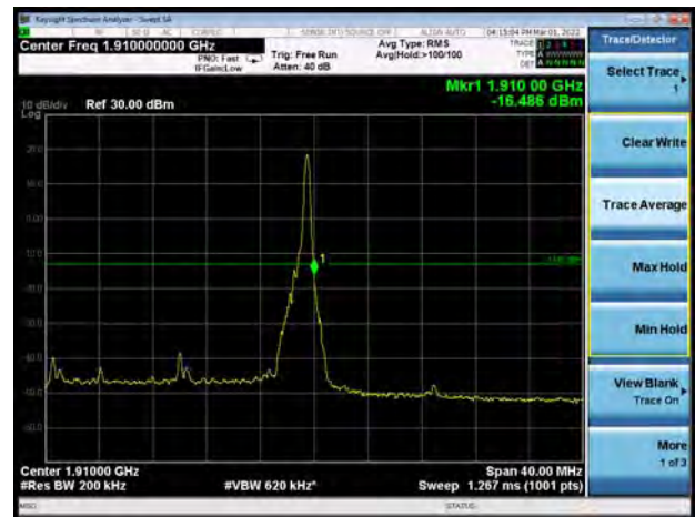
DC_12A_n2A 64QAM 20MHz CH-High 100%RB
