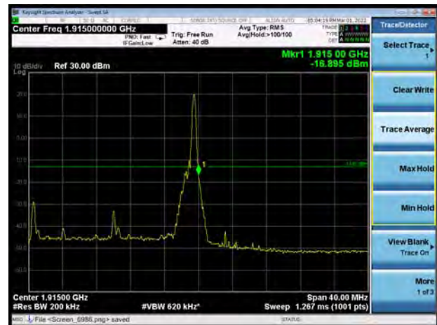
NR n25 P1/2 BPSK 20MHz CH-High 100%RB
