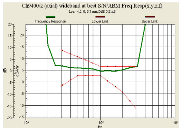
Fig. 7.8 WCDMA Band II Ch9400
