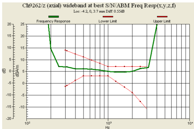
Fig. 7.7 WCDMA Band II Ch9262
