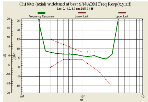
Fig 7.2 GSM850 Ch189
