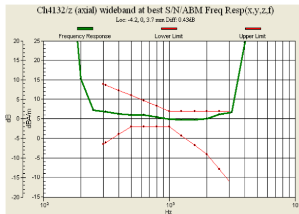
Fig. 7.10 WCDMA Band V Ch4132
