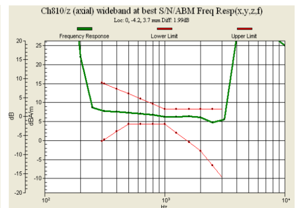
Fig 7.6 GSM1900 Ch810
