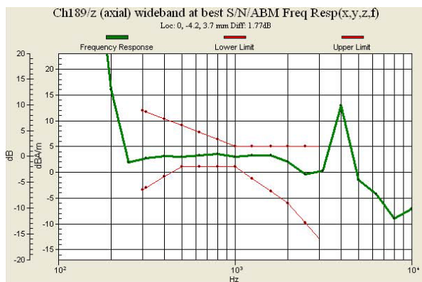
Fig 7.1 GSM850 Ch189
