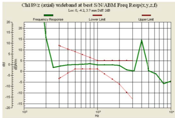
Fig 7.1 GSM850 Ch189
