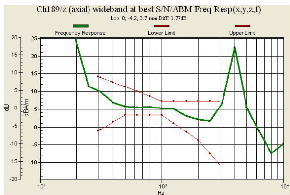
Fig 7.1 GSM850 Ch189
