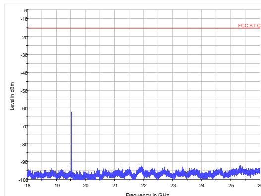
GFSK-CH78 18GHz~26.5GHz
