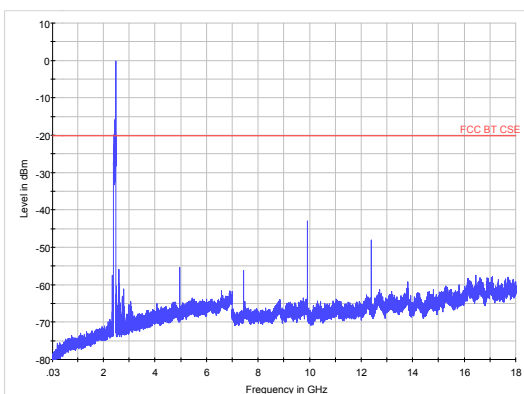
GFSK-CH78 30MHz~18GHz
