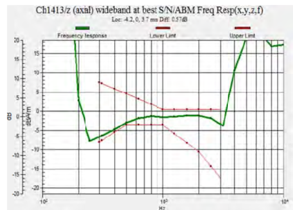
Fig. 7.9 WCDMA Band IV Ch1413
