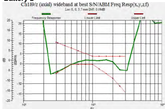
Fig 7.1 GSM850 Ch189
