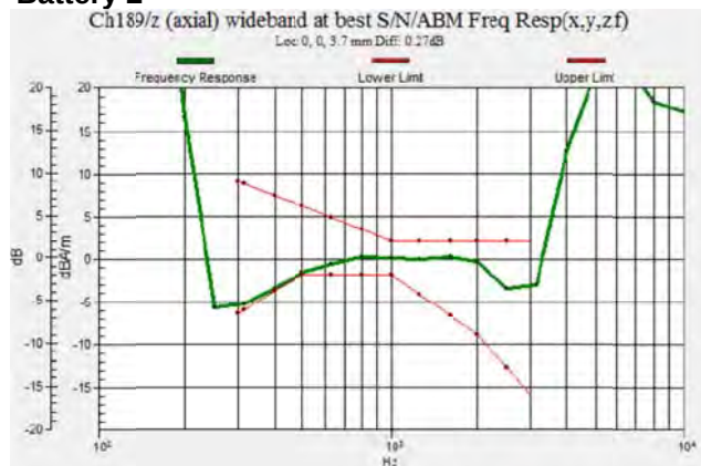
Fig 7.6 GSM850 Ch189
