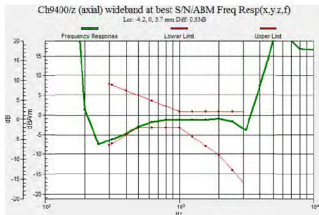
Fig. 7.10 WCDMA Band II Ch9400
