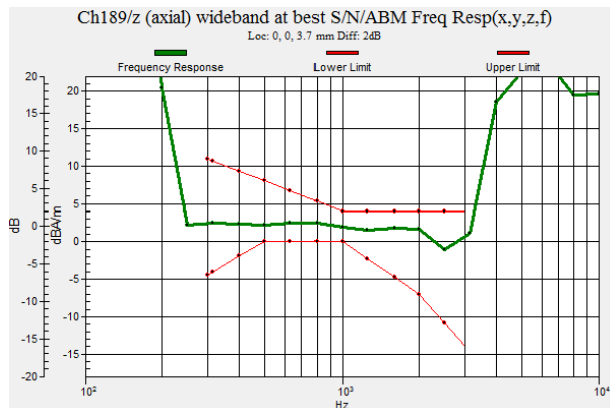
Fig 7.1 GSM850 Ch189
