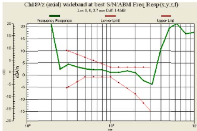
Fig 7.1 GSM850 Ch189
