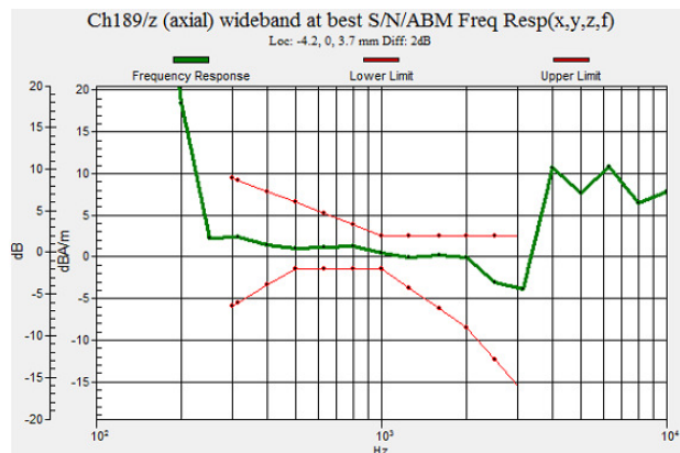
Fig 7.1 GSM850 Ch189
