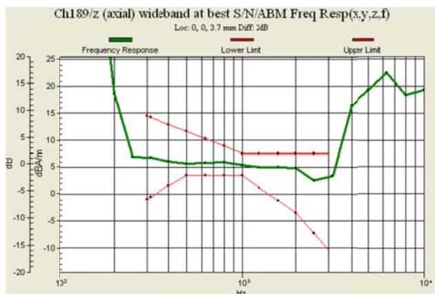
Fig 7.1 GSM850 Ch189
