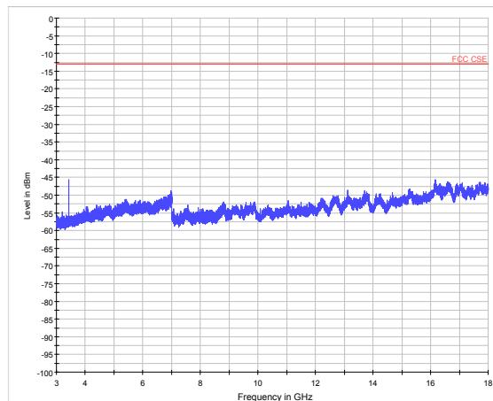
NB-IOT Band 4 15KHz CH-Middle 3GHz~18GHz
