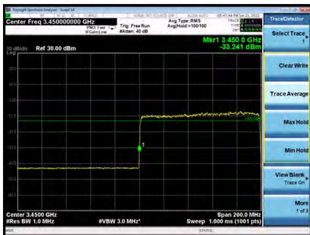
DC_5A-n78A (Subset 1) 256QAM 100MHz CH-Low 1RB
