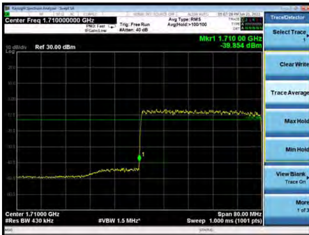
DC_2A-n66A 16QAM 20MHz CH-Low 100%RB
