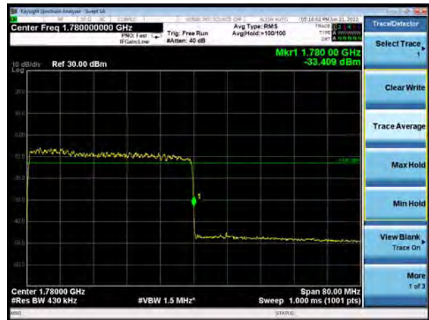
DC_2A-n66A 16QAM 20MHz CH-High 100%RB
