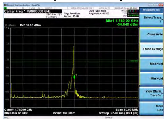
NR n66 QPSK 20MHz CH-High 1RB
