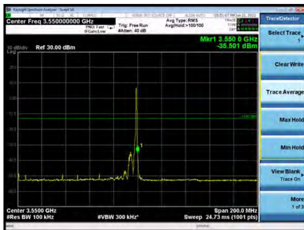
DC_5A-n78A (Subset 1) 64QAM 100MHz CH-High 100%RB
