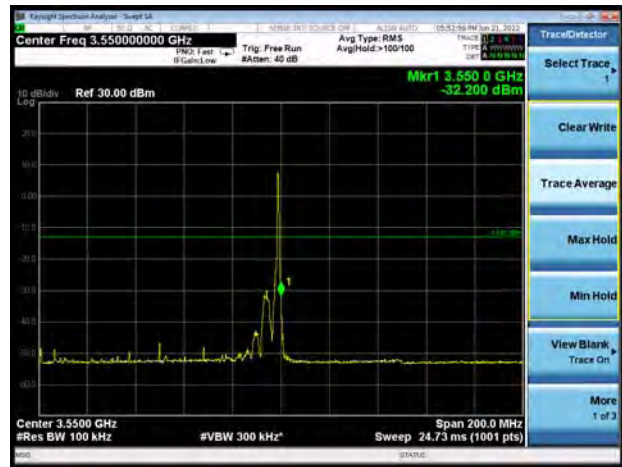
DC_5A-n78A (Subset 1) P1/2 BPSK 100MHz CH-High 100%RB
