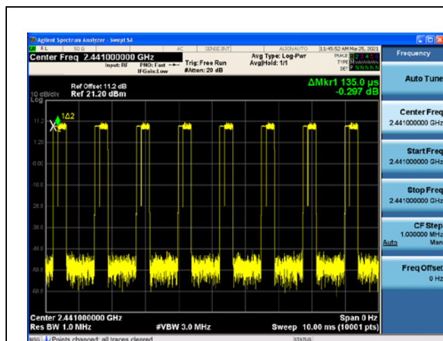
Modulation: \pi/4 DQPSK DH1 2441
