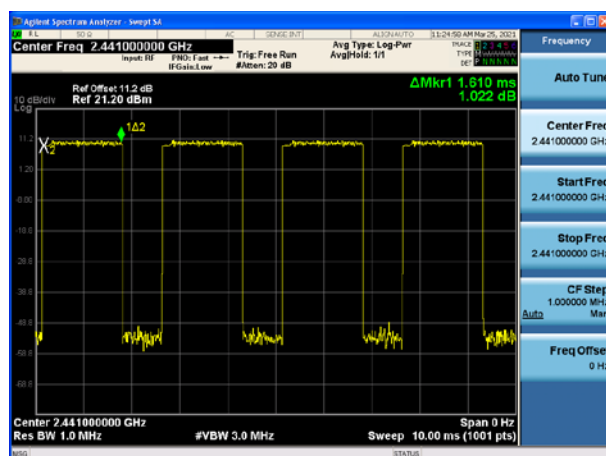
Modulation: \pi/4 DQPSK DH3 2441
