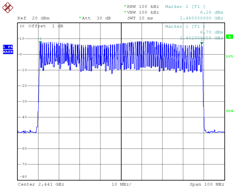
(Plot A: GFSK)
