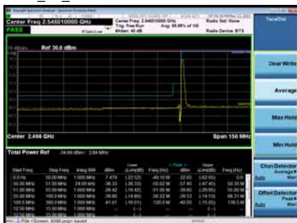
DC 2A n41A 100MHz QPSK 1RB CH-Low
