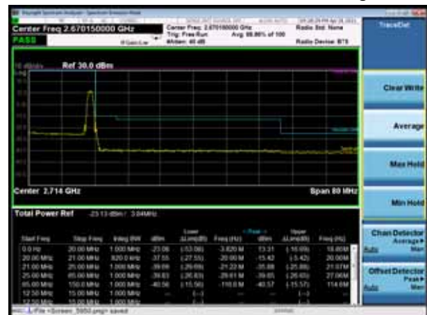
NR n41 40MHz 64QAM 100%RB CH-High
