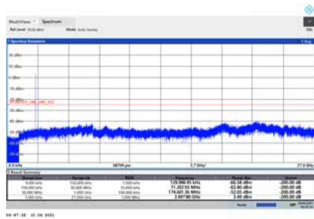
NR n41 QPSK 40MHz CH-Middle
