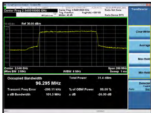
NR n41 P1/2 BPSK 100%RB 100MHz CH-Middle
