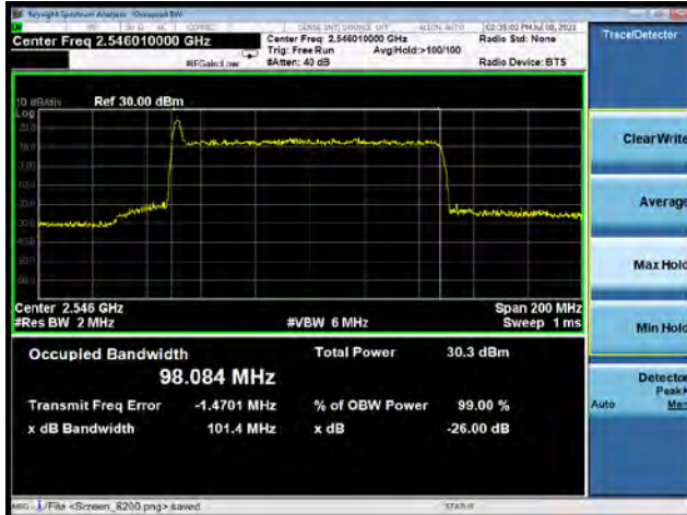
DC_66A-n41A 64QAM 100%RB 100MHz CH-Middle
