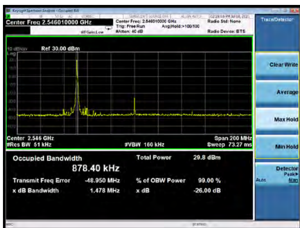
DC_66A-n41A 64QAM 1%RB 100MHz CH-Middle
