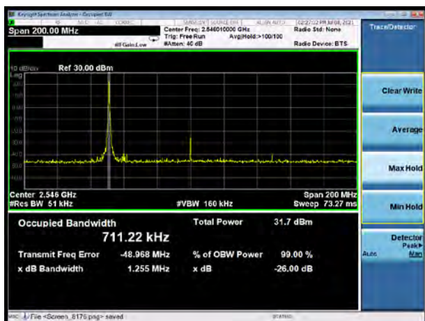
DC_66A-n41A 16QAM 1%RB 100MHz CH-Middle
