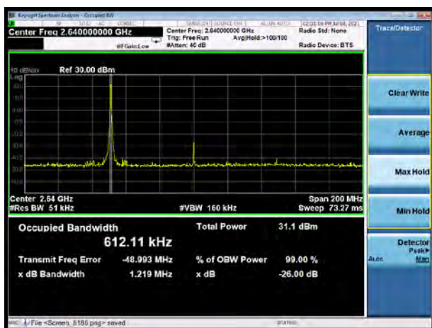
DC_66A-n41A 16QAM 1%RB 100MHz CH-High
