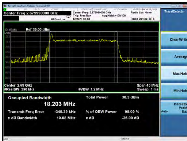
DC_66A-n41A 64QAM 100%RB 20MHz CH-High
