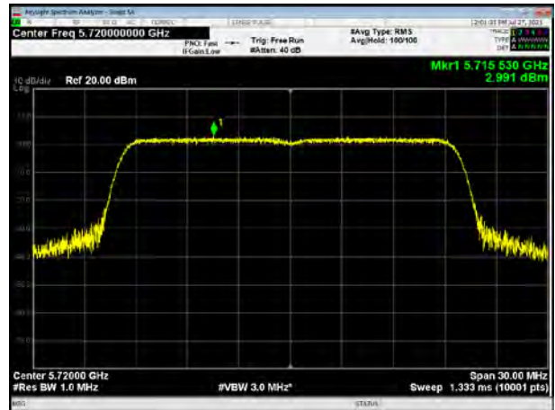
802.11ax HE20 242Tone: 5720
