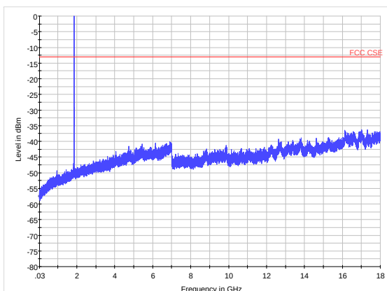
GSM 1900 CH-Middle 30MHz~18GHz
