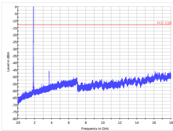
WCDMA Band II CH-Middle 30MHz~18GHz
