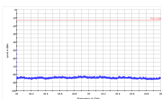
GSM 1900 CH-Middle 18GHz~20GHz
