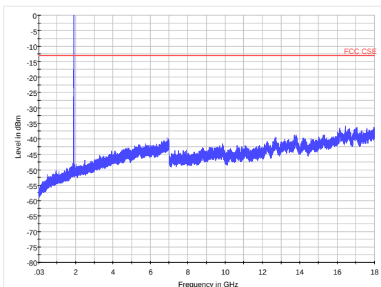
GSM 1900 CH-High 30MHz~18GHz
