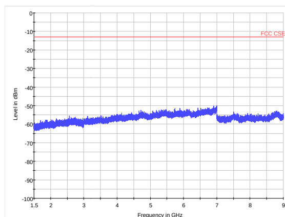
LTE Band 12 10MHz CH23095 1.5GHz~9GHz
