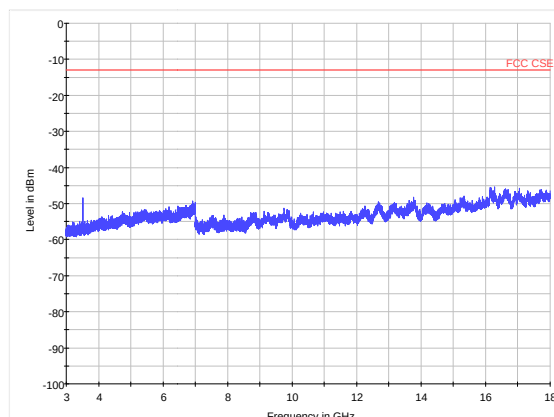
LTE Band 4 CH20393 3GHz~18GHz
