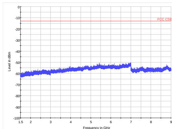
LTE Band 12 5MHz CH23095 1.5GHz~9GHz
