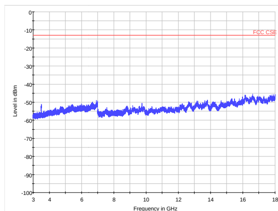
LTE Band 4 CH20375 3GHz~18GHz
