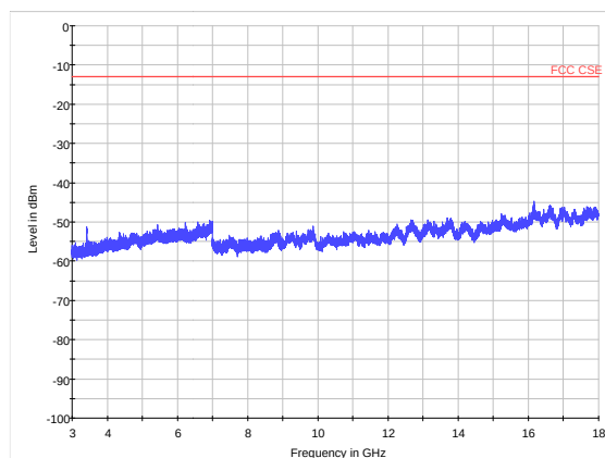
LTE Band 4 CH19965 3GHz~18GHz
