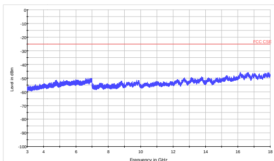
LTE Band 7 10MHz CH21100 3GHz~18GHz
