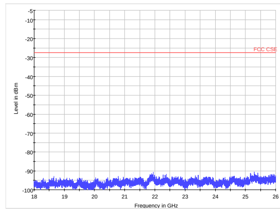
BLE CH39 18GHz to 26GHz
