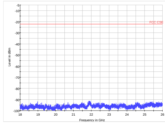
BLE CH19 18GHz to 26GHz
