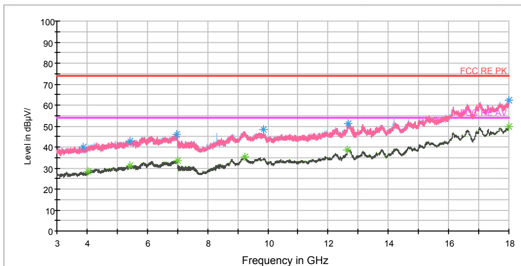
RE 3-18GHz PK+AV_BELL SWEEP
