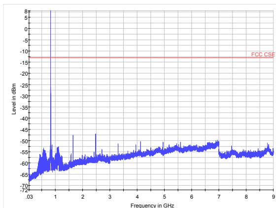
GSM 850 CH-Low 30MHz~9GHz
