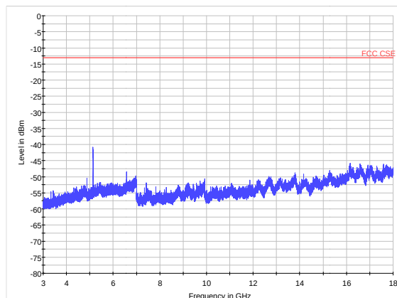
WCDMA Band IV CH-Middle 3GHz ~18GHz
