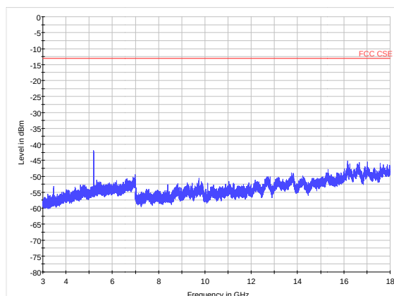
WCDMA Band IV CH-High 3GHz ~18GHz
