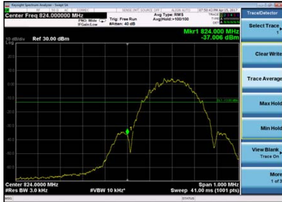
GSM 850 EGPRS CH-Low
