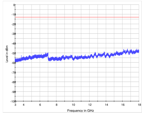
LTE Band 2 5MHz CH-Middle 3GHz~18GHz
