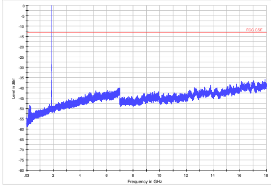
GSM 1900 CH-Middle 30MHz~18GHz
