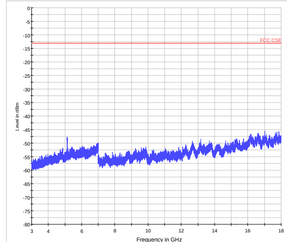
WCDMA Band IV CH-Middle 3GHz ~18GHz
