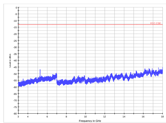
WCDMA Band IV CH-High 3GHz ~18GHz
