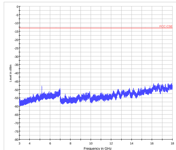
WCDMA Band IV CH-High 3GHz ~18GHz
