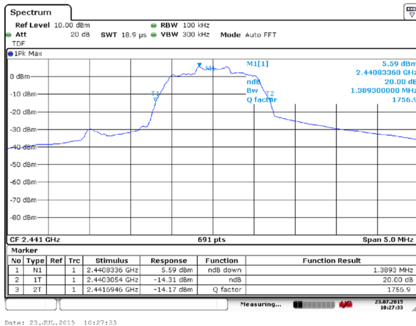
Fig. 54 Occupied 20dB Bandwidth ( \pi/4 DQPSK, Ch 39)
