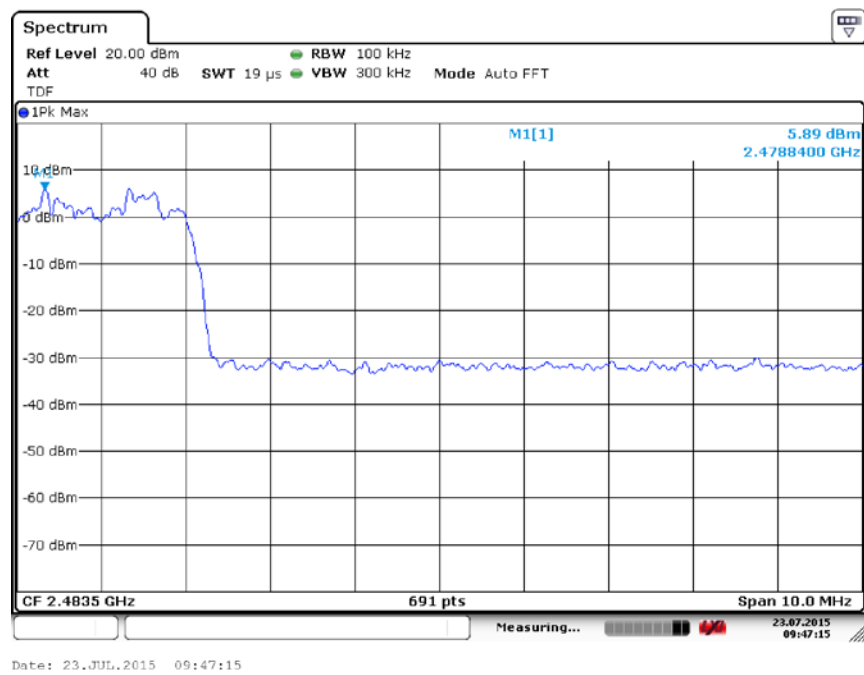
Fig. 13 Band Edges ( \pi/4 DQPSK, Ch 78, Hopping ON)
