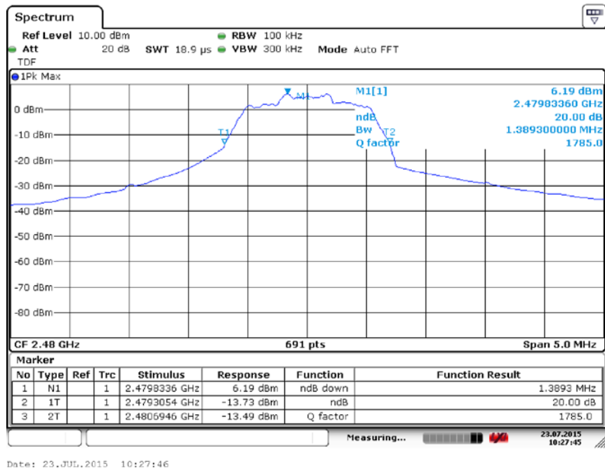
Fig. 55 Occupied 20dB Bandwidth ( \pi/4 DQPSK, Ch 78)
