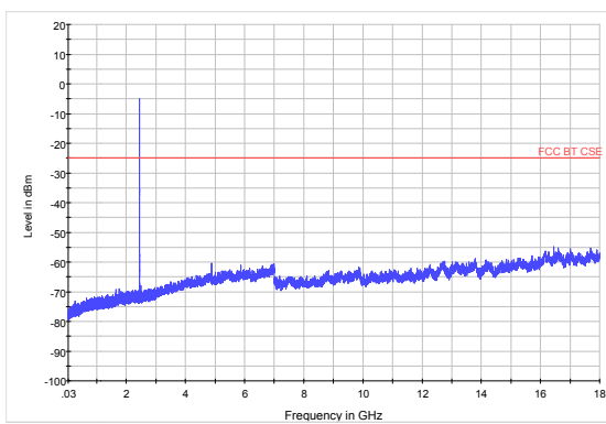
EDR-CH78 30MHz to 18GHz
