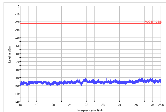
GFSK-CH78 18GHz to 26.5GHz
