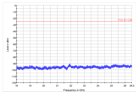
EDR-CH78 18GHz to 26.5GHz
