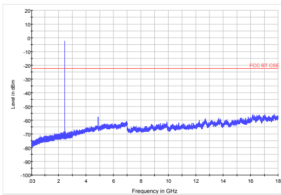
GFSK-CH78 30MHz to 18GHz
