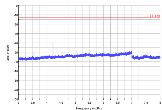
LTE Band 12 10MHz CH-Middle 3GHz~8GHz
