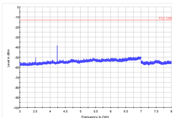
LTE Band 13 10MHz CH-Middle 3GHz~8GHz
