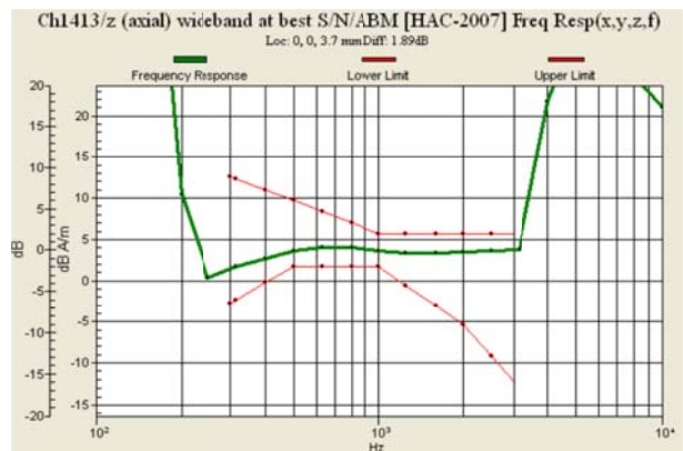
Fig 9.4 WCDMA Band IV Ch1413
