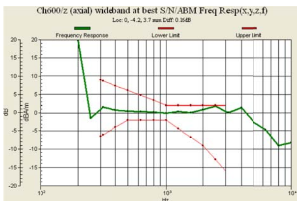
Fig 7.3 CDMA2000 BC1 Ch600
