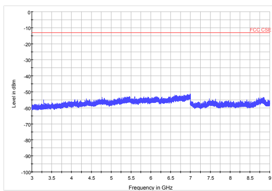
LTE Band 5 5MHz CH20425 3GHz~9GHz
