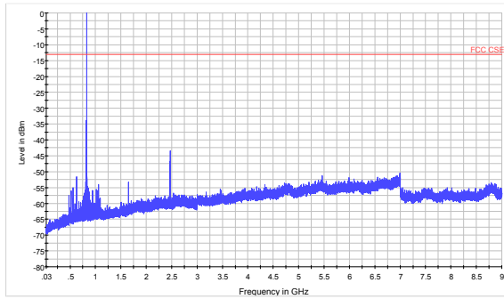
GSM 850 CH128 30MHz~9GHz
