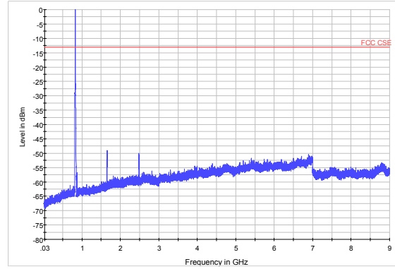
WCDMA Band V CH4183 30MHz~9GHz
