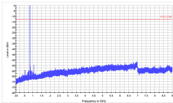
GSM 850 CH251 30MHz~9GHz
