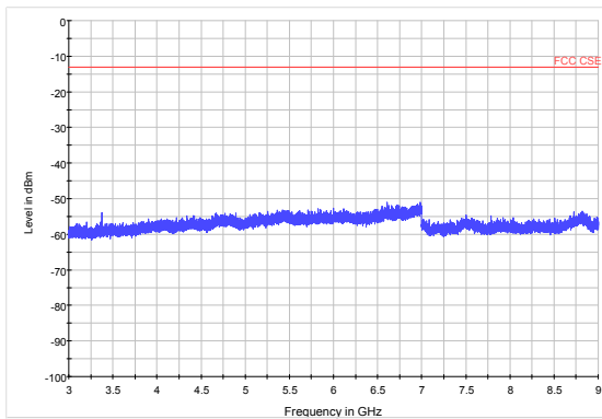
LTE Band 5 10MHz CH20600 3GHz~9GHz
