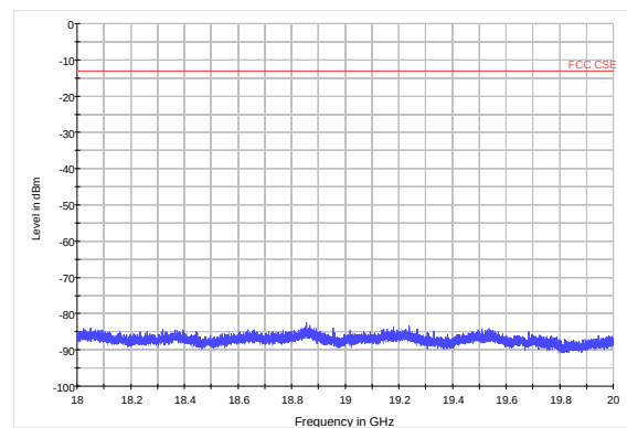
LTE Band 25 20MHz CH26140 18GHz~20GHz
