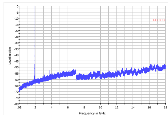
WCDMA Band II CH9262 30MHz~18GHz
