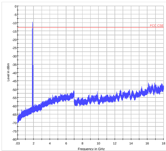
CDMA BC1 1xRTT CH600 30MHz~18GHz
