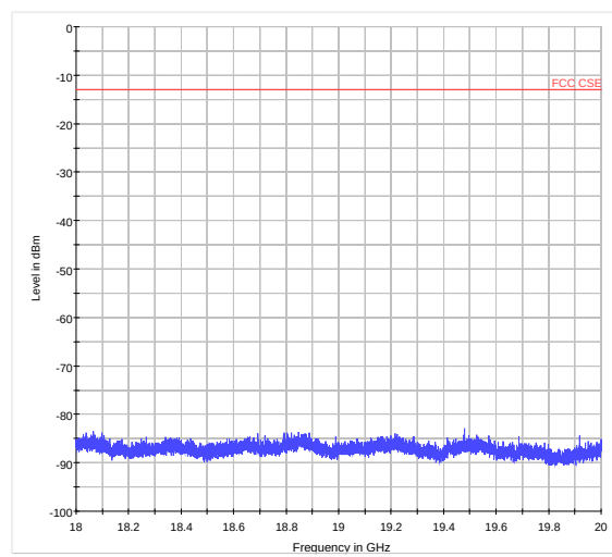
CDMA BC1 1xRTT CH600 18GHz~20GHz
