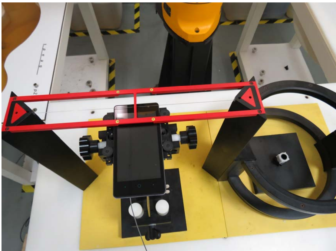
HAC T-coil
