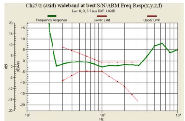
Fig 8.4 CDMA2000 BC1 Ch25
