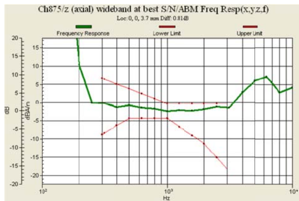
Fig. 8.9 CDMA2000 BC15 Ch875
