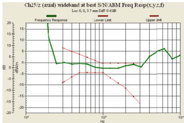
Fig. 8.7 CDMA2000 BC15 Ch25
