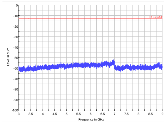
LTE Band 12 CH23095 3GHz~9GHz
