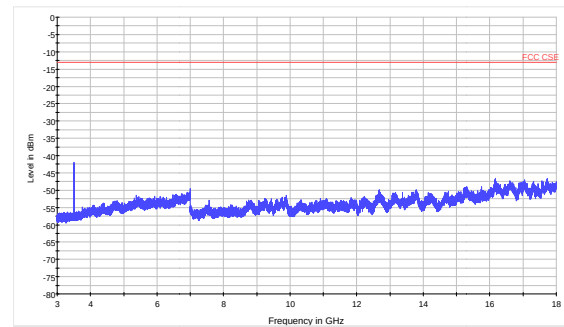
WCDMA Band IV Channel1513 3GHz ~18GHz
