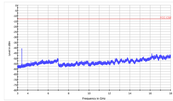
WCDMA Band IV Channel1312 3GHz ~18GHz
