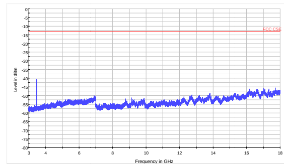
WCDMA Band IV Channel1413 3GHz ~18GHz
