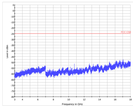
LTE Band 41 CH41565 3GHz~18GHz
