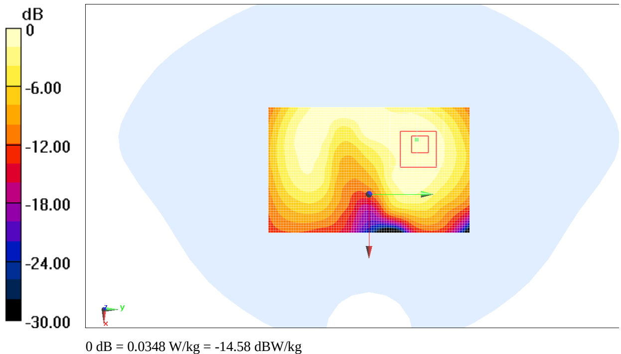
Fig. 6 2450 MHz CH11
