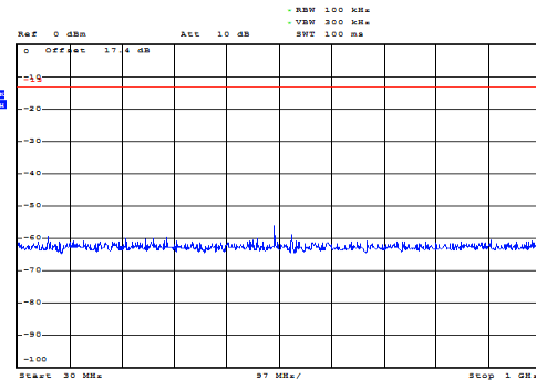
GSM 1900 CH-Middle 30MHz~1GHz
