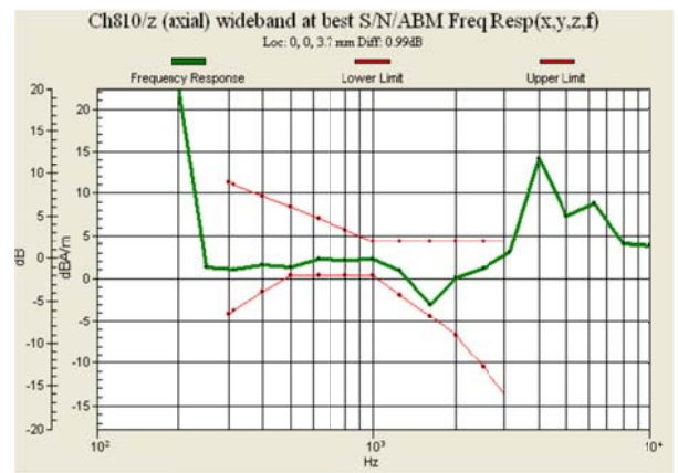
Fig 7.6 GSM1900 Ch810
