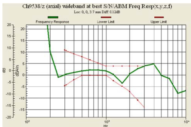
Fig. 7.15 WCDMA Band II Ch9538
