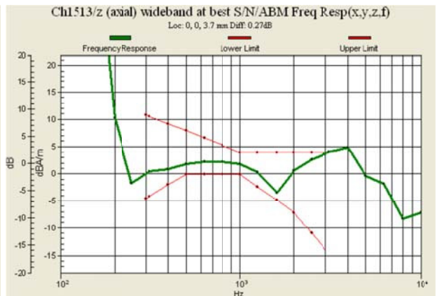
Fig. 7.12 WCDMA Band IV Ch1513
