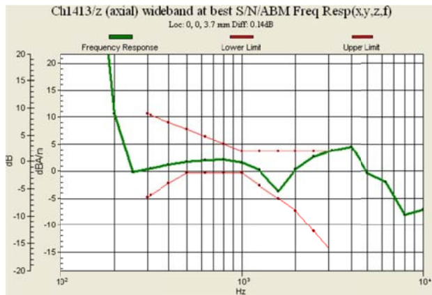
Fig. 7.11 WCDMA Band IV Ch1413
