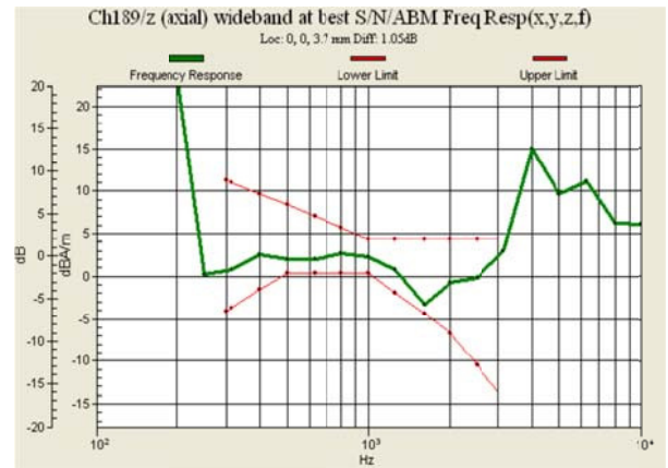
Fig 7.2 GSM850 Ch189
