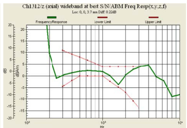
Fig. 7.10 WCDMA Band IV Ch1312
