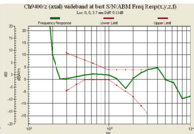
Fig. 7.14 WCDMA Band II Ch9400
