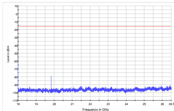
EDR-CH78 18GHz to 26.5GHz
