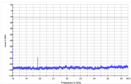
GFSK-CH78 18GHz to 26.5GHz
