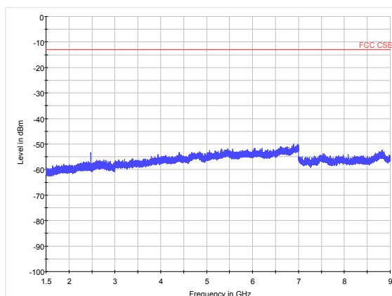
LTE Band 26 10MHz CH-Middle 1.5GHz~9GHz
