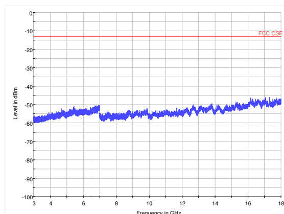
LTE Band 41 20MHz CH41140 3GHz~18GHz
