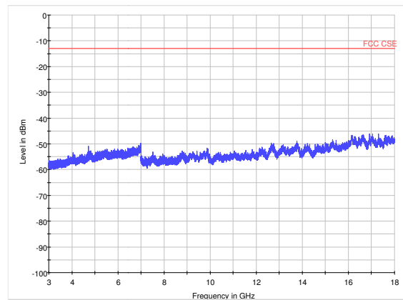
LTE Band 41 10MHz CH41185 3GHz~18GHz
