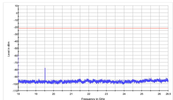
BLE CH19 18GHz to 26.5GHz
