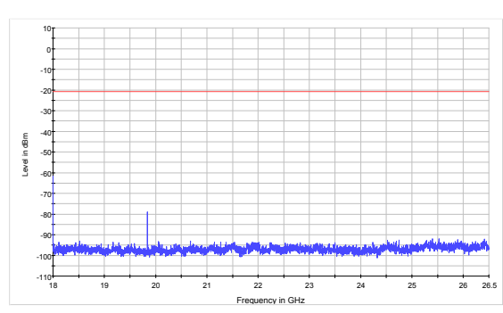
BLE CH39 18GHz to 26.5GHz
