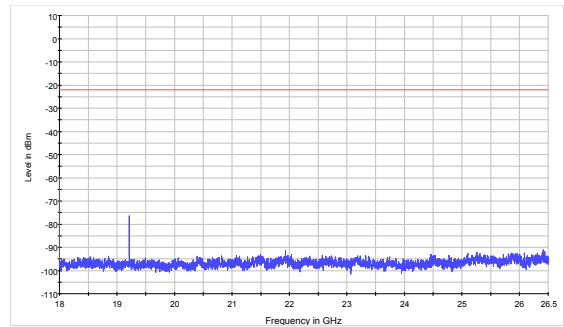
BLE CH0 18GHz to 26.5GHz
