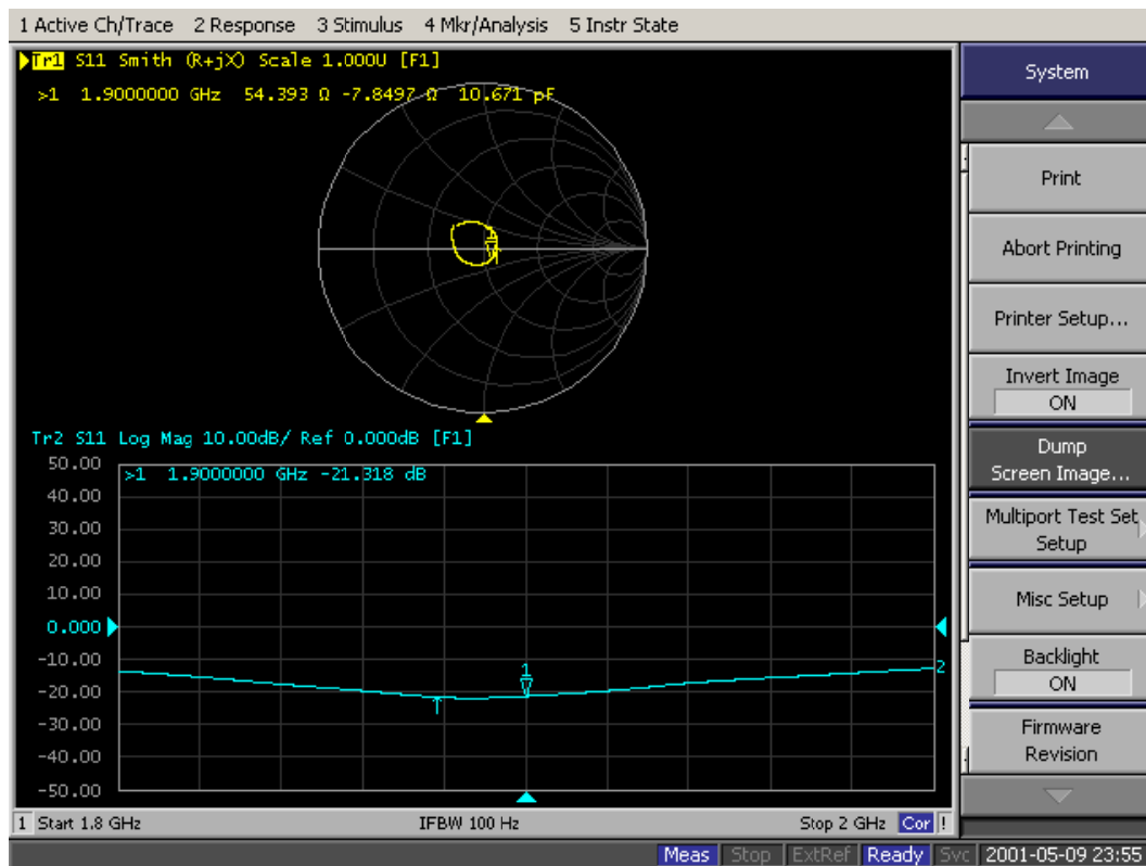
Dipole D1900V2-5/4/2016
