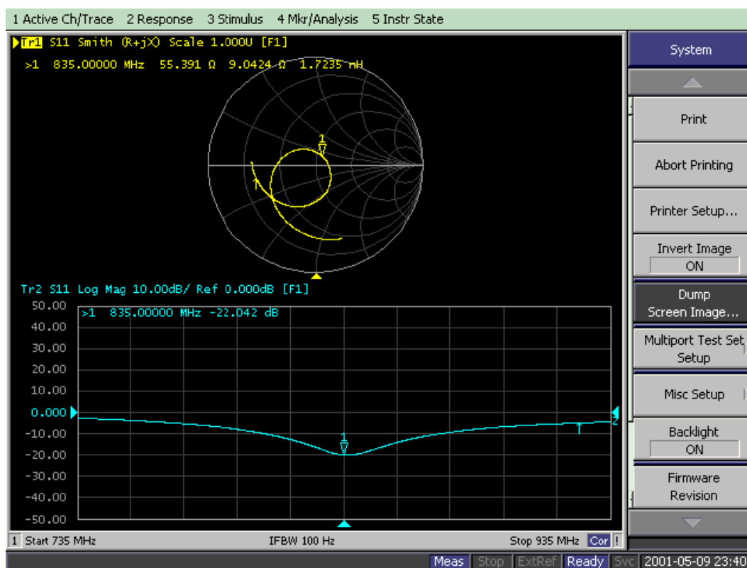
Dipole D835V2-5/4/2016
