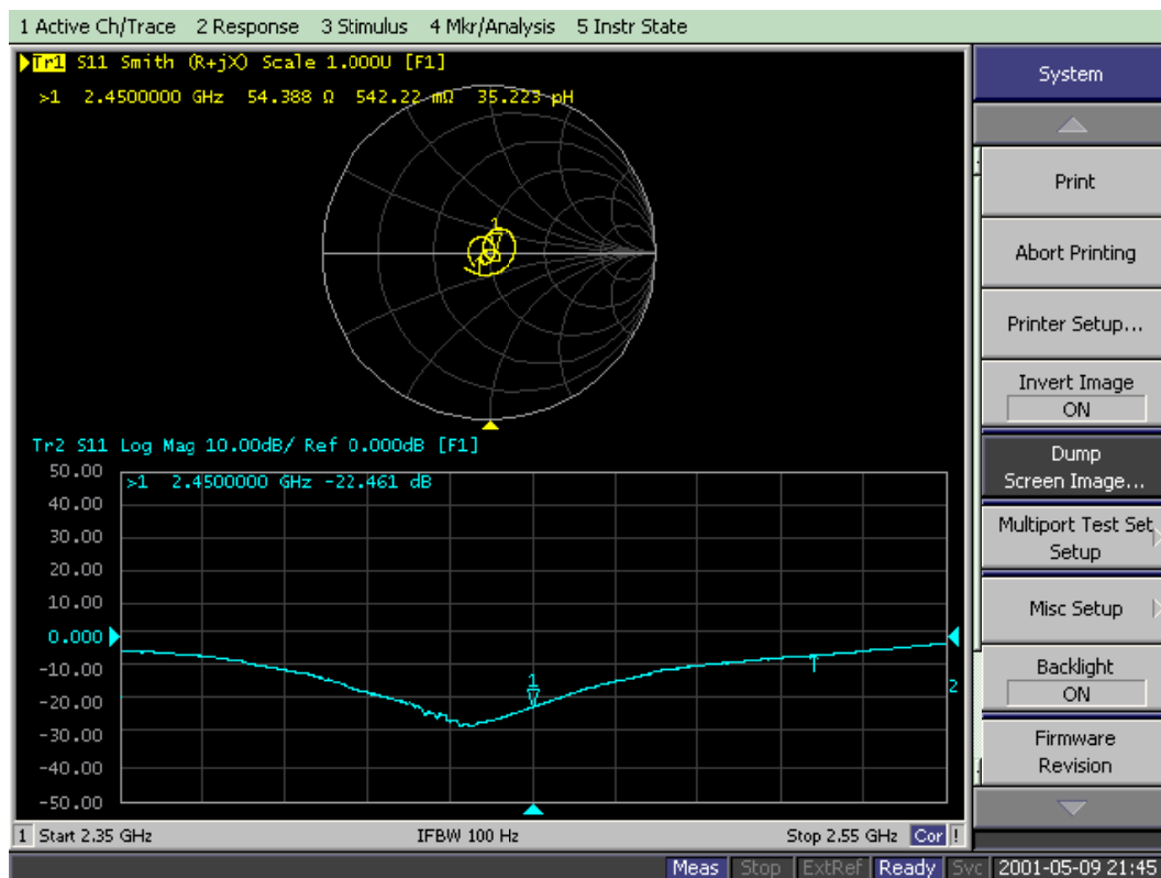
Dipole D2450V2-5/4/2016
