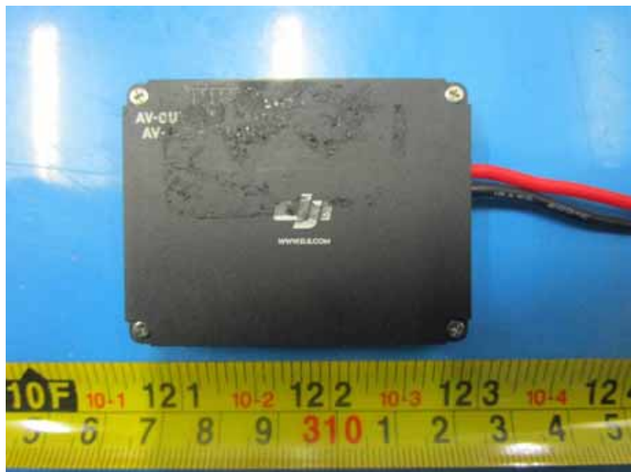
EUT –Display Module Bottom View
