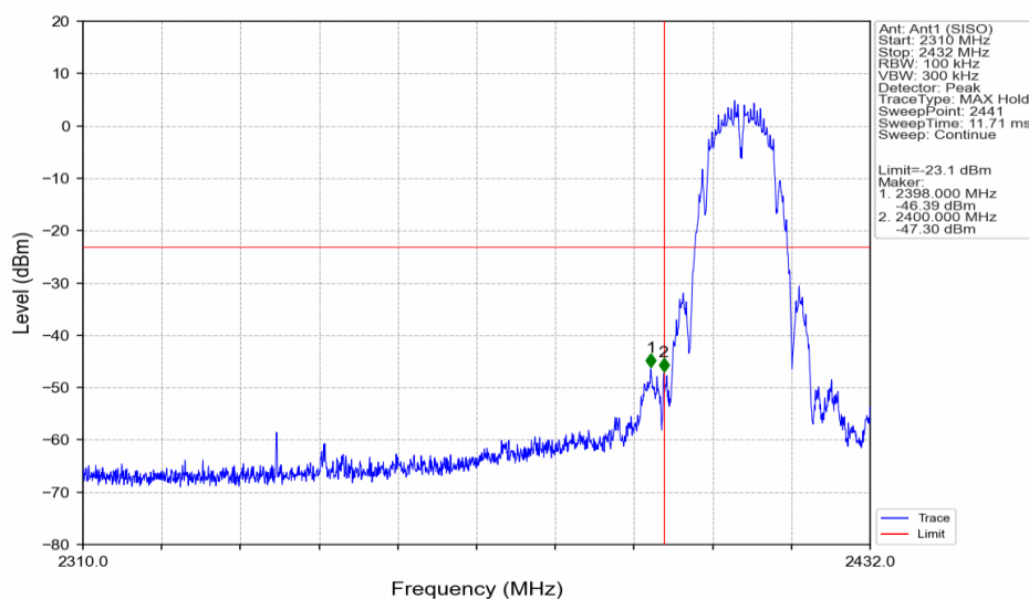
802.11b_LCH_2412MHz_Ant1 (SISO)_NTNV
