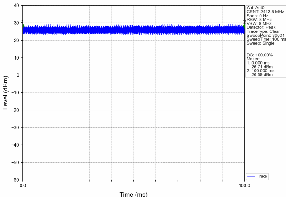
20M_LCH_2412.5MHz_Ant0_NTNV
